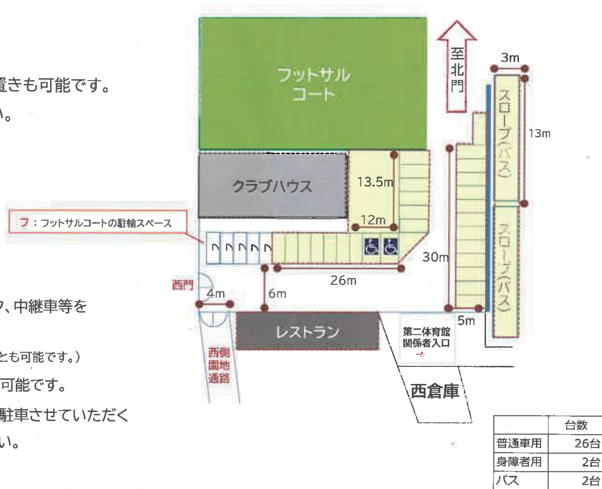
第二体育館専用駐車場見取り図
